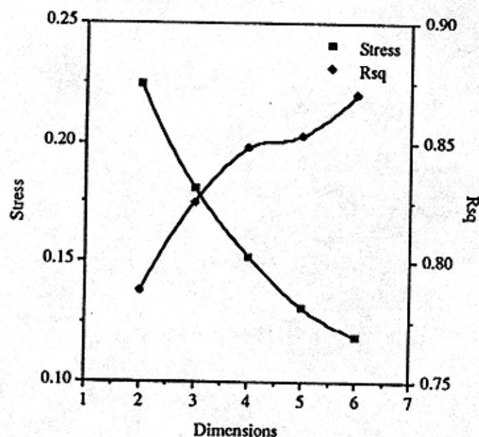
Figure 2. Stress et proportion de variance expliquée (Rs q ) pour les analyses INDSCAL (2 à 6 dimensions) sur les matrices de distances entre atteintes aux droits de l'homme.
